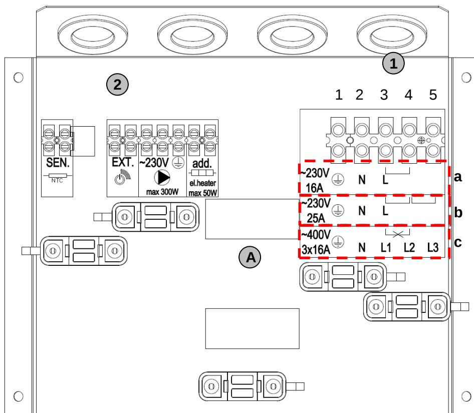
Abbildung 14: Elektrische Anschlüsse
