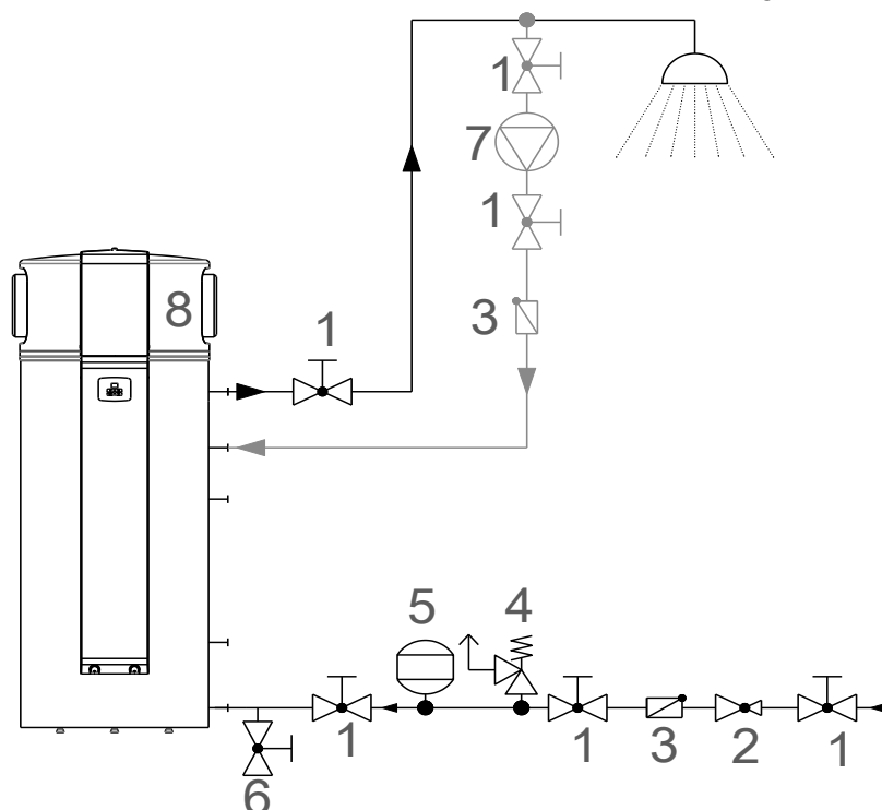
Abbildung 7: Anschluss ans Wasserversorgungsnetzwerk
