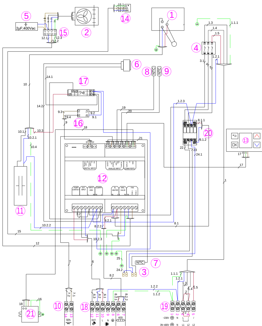
Abbildung 15: Elektrischer Schaltplan
