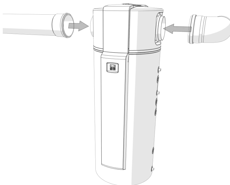
Abbildung 8: Luftkanalanschluss
