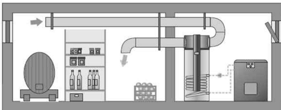
Abbildung 3: Ansaugen und Ausblasen aus einem Nebenraum (Nebenraumkühlung)
