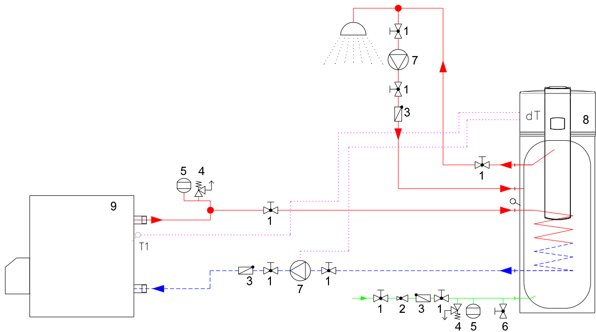
Bild 7: Gerät in Kombination mit Warmwasserspeicher
