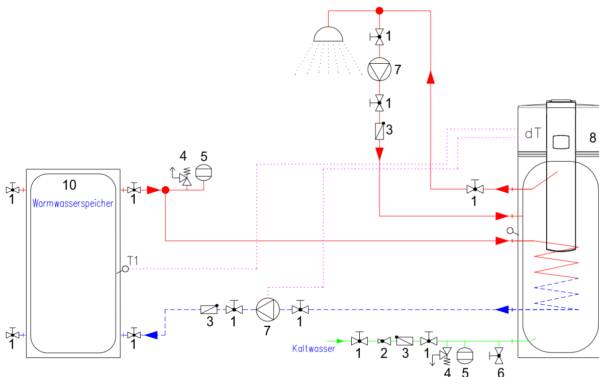
Bild 5: Gerät in Kombination mit einem Kessel
