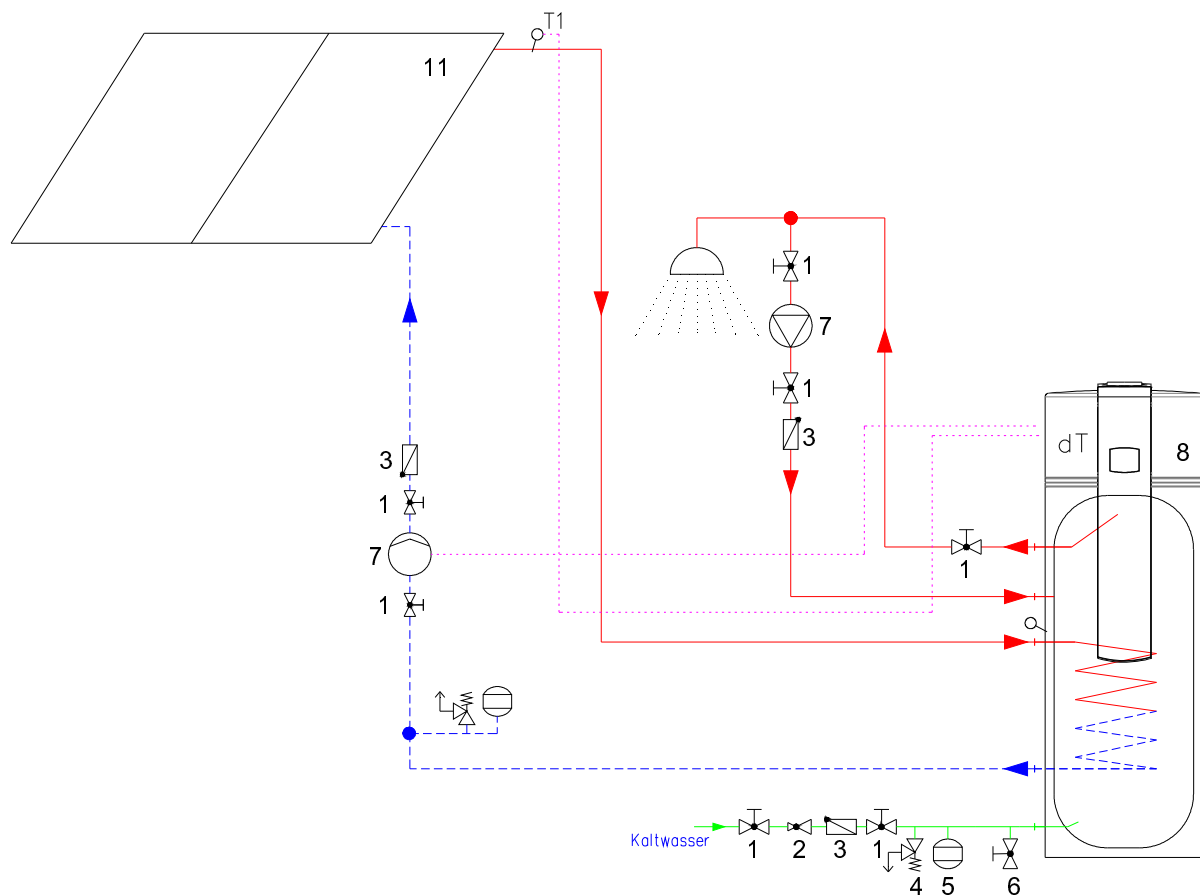
Bild 6: Gerät in Kombination mit Sonnenkollektoren
