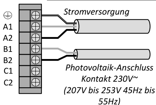
Schema Eingang Potential 230V
