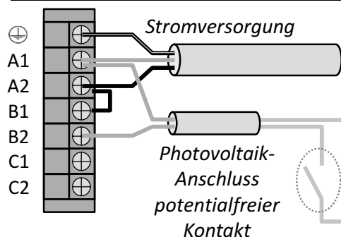
Schema Eingang potentialfreier Kontakt
