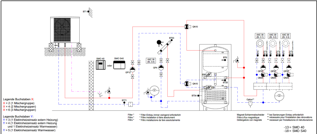
Funktionsschema 8.2
